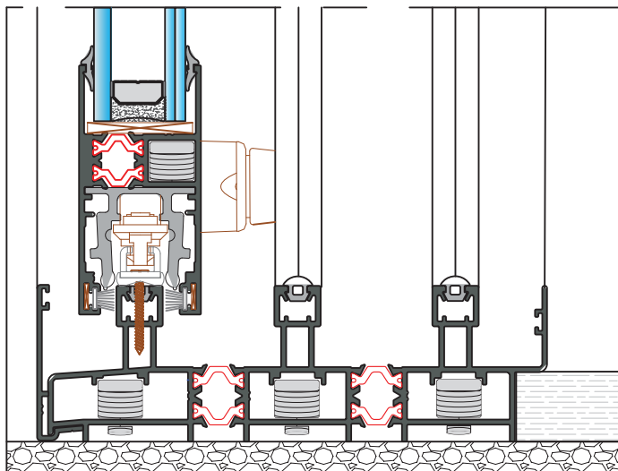
CORTE 16
