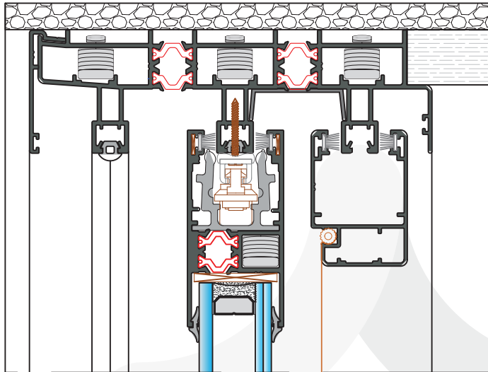
CORTE 18
