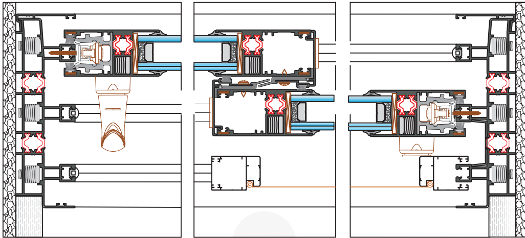
CORTE 13
