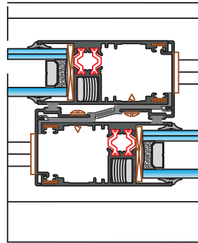
CORTE 9
