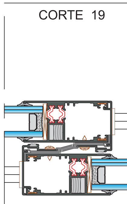
Janela / Sacada correr 2 folhas
