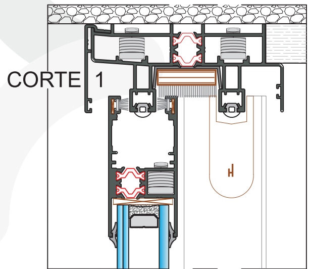
Janela/Sacada correr 2 folhas
