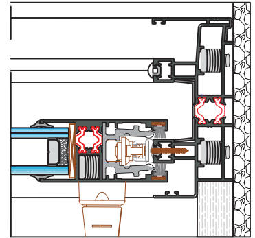
CORTE 10
