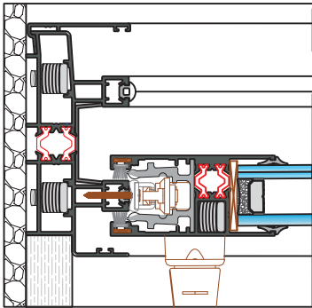
CORTE 8
