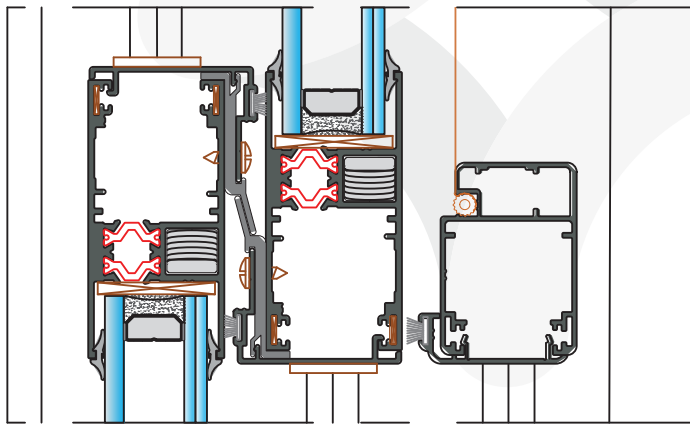
CORTE 17
