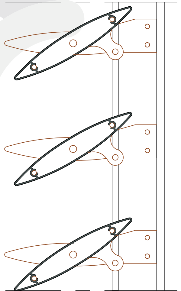
CORTE 1
